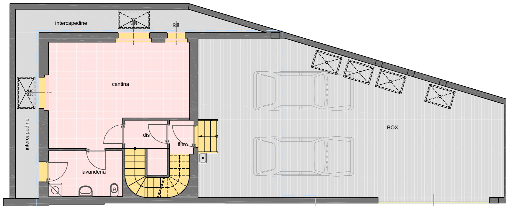
INTERRATO
